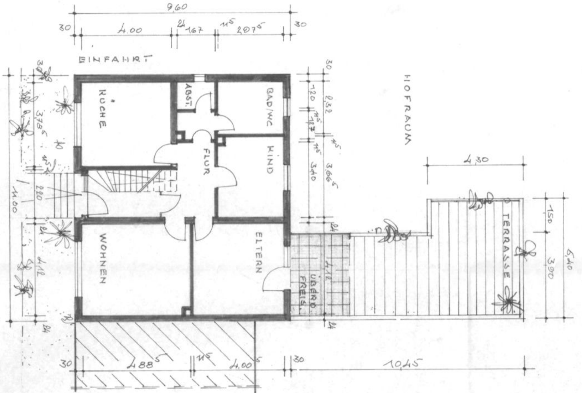
Erdgeschoss
